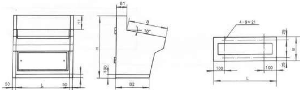
盘底与基础安装尺寸示意图
