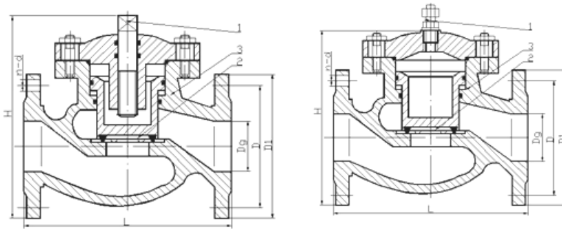
YF 型油阀结构图
